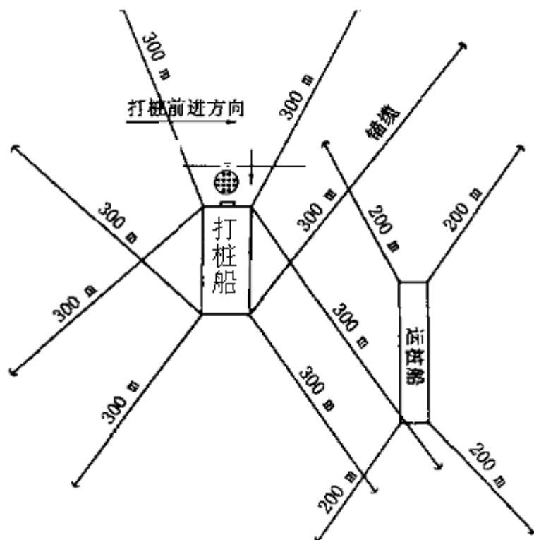
图 1.4-2 打桩船与驳船抛锚定位示意图
