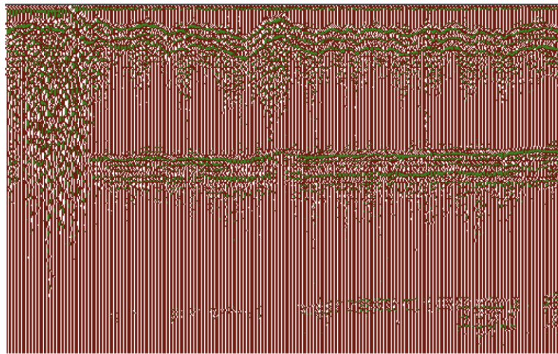
图 2.2-9 正极性反射特征（西部区域，S-N 方向）
