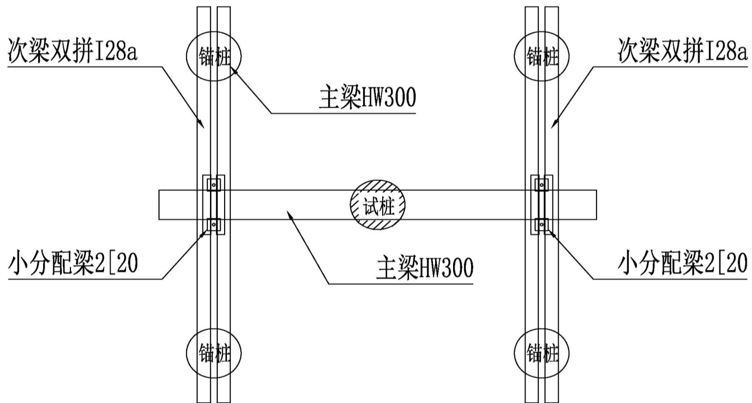
锚桩横梁反力装置示意图
