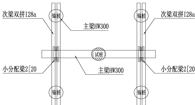
图 1.3-2 锚桩横梁反力装置示意图
