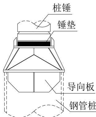
图 1.4-3 钢管桩锤击沉桩吊钟式替打示意图
